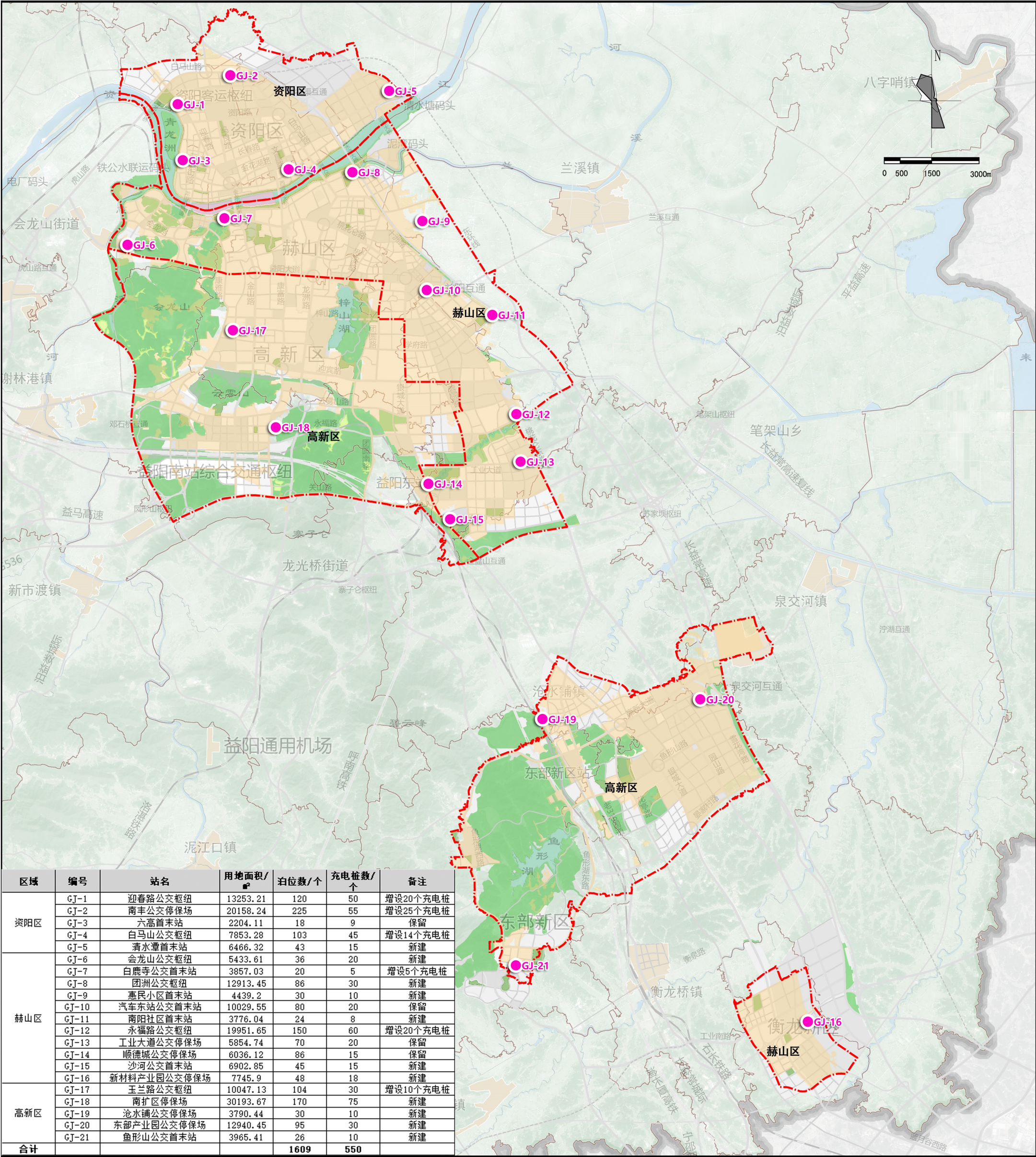
公交车专用充电设施规划图
